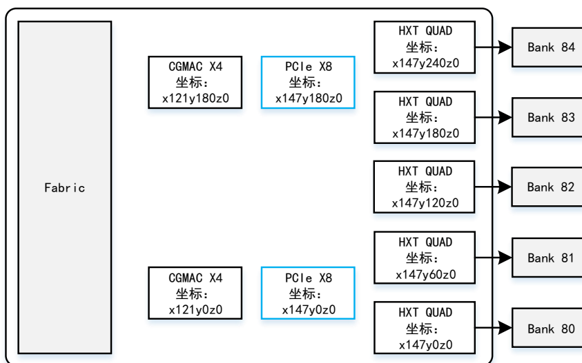
图 1-2 PH2A106FLG900 器件中的 PCIe Express 控制器和 PHY 资源示意图
