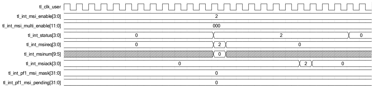
图 2-30 PF1 发送 MSI 中断
