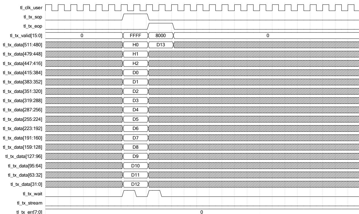
图 2-8 发送 3DW Header With 14DW Payload
