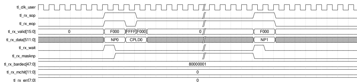
图 2-16 接收 Non-Posted TLP 报文
