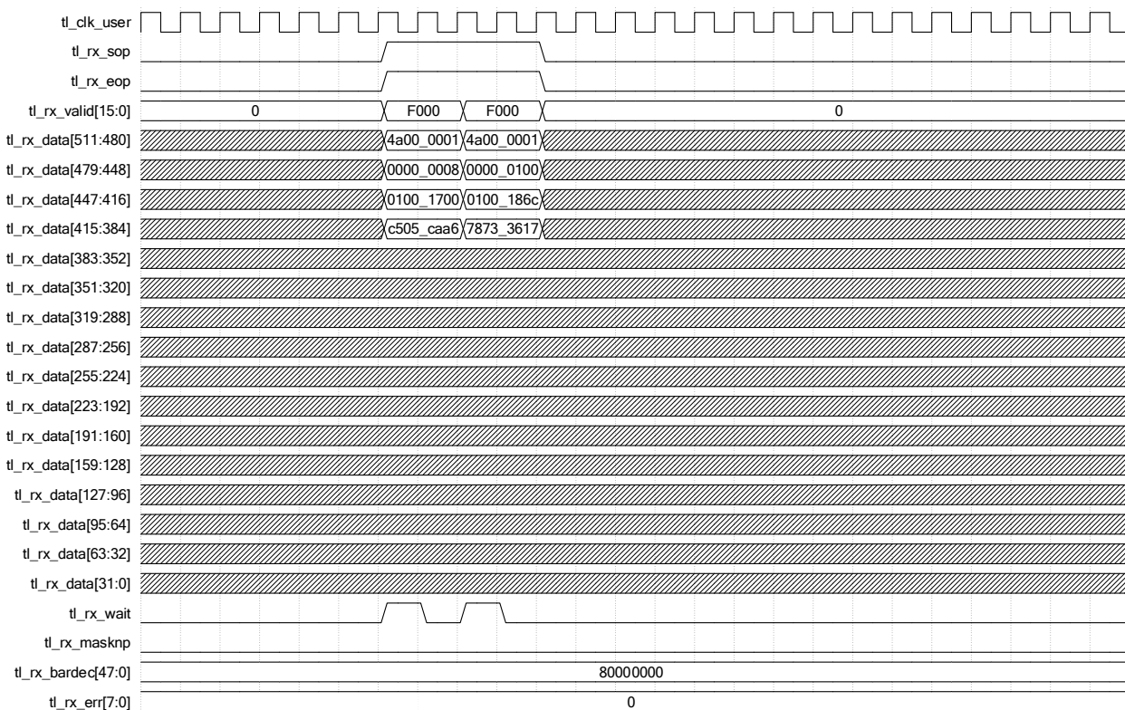
图 2-21 连续接收两次 CPLD
