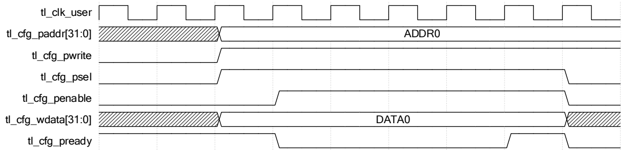
图 2-23 写操作有等待
