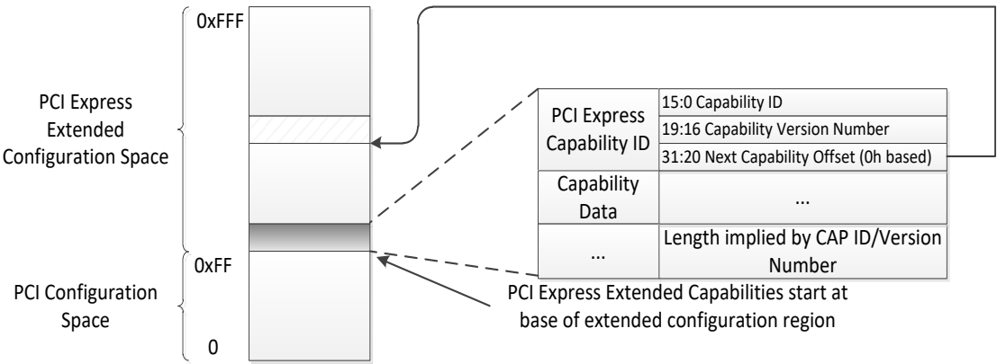
图 1-5 PCI Express 扩展配置空间地址分配
