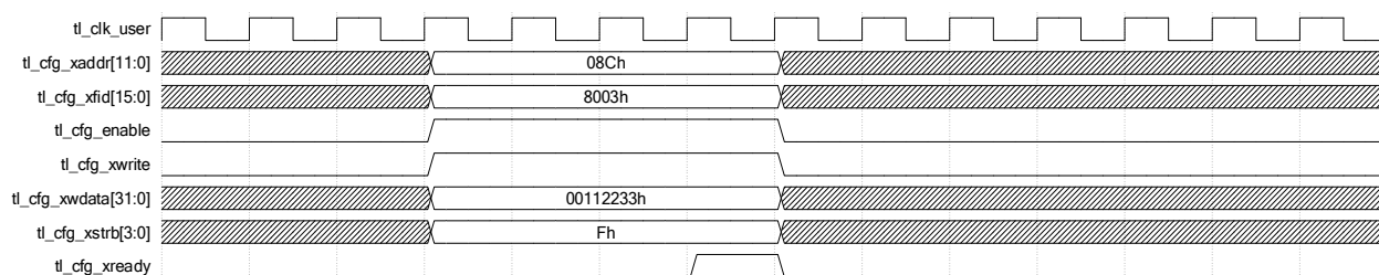
图 2-35 对 PF 进行写操作
