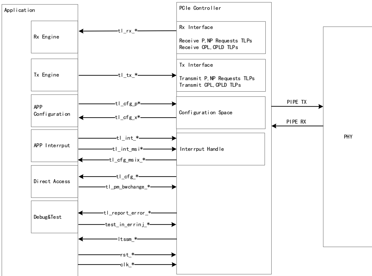
图 2-1 PCI Express 控制器接口信号
