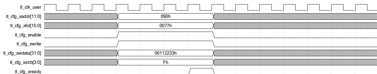
图 2-37 对 VF 进行写操作
