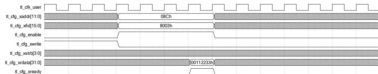
图 2-36 对 PF 进行读操作
