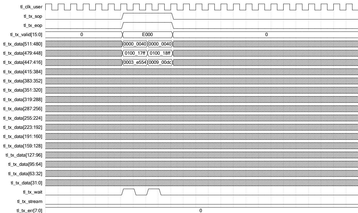
图 2-10 连续发送两次读请求
