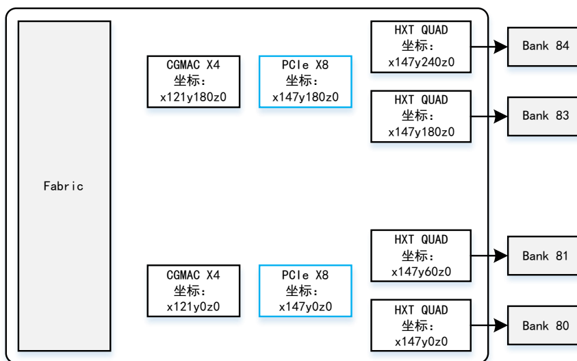
图 1-1 PH2A106FLG676 器件中的 PCIe Express 控制器和 PHY 资源示意图
