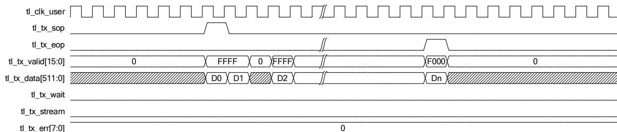
图 2-5 发送过程 valid 信号置 0
