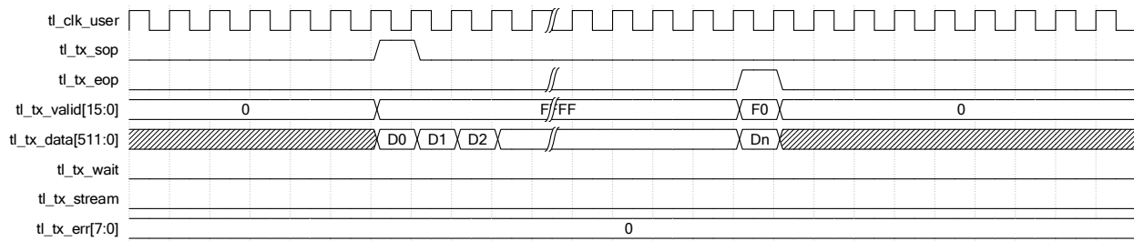
图 2-3 发送过程 wait 信号没有反压
