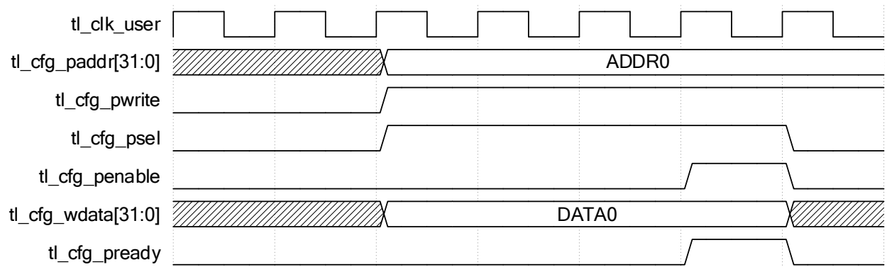
图 2-22 写操作无等待
