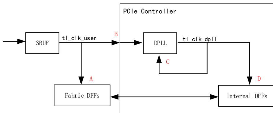
图 3-3 PCIe 控制器内外时钟结构
