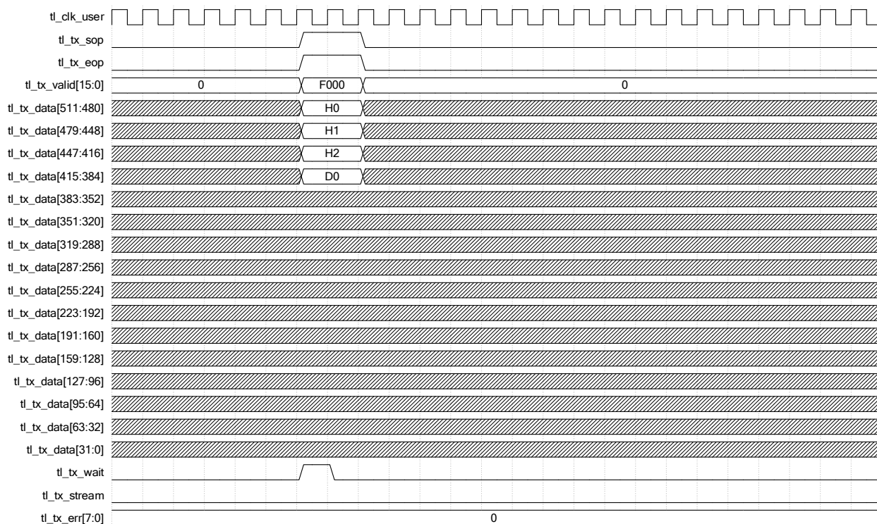
图 2-7 发送 3DW Header With 1DW Payload
