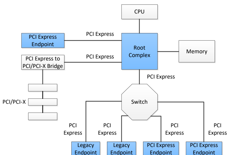
图 1-3 PCI Express 系统结构拓扑图示例
