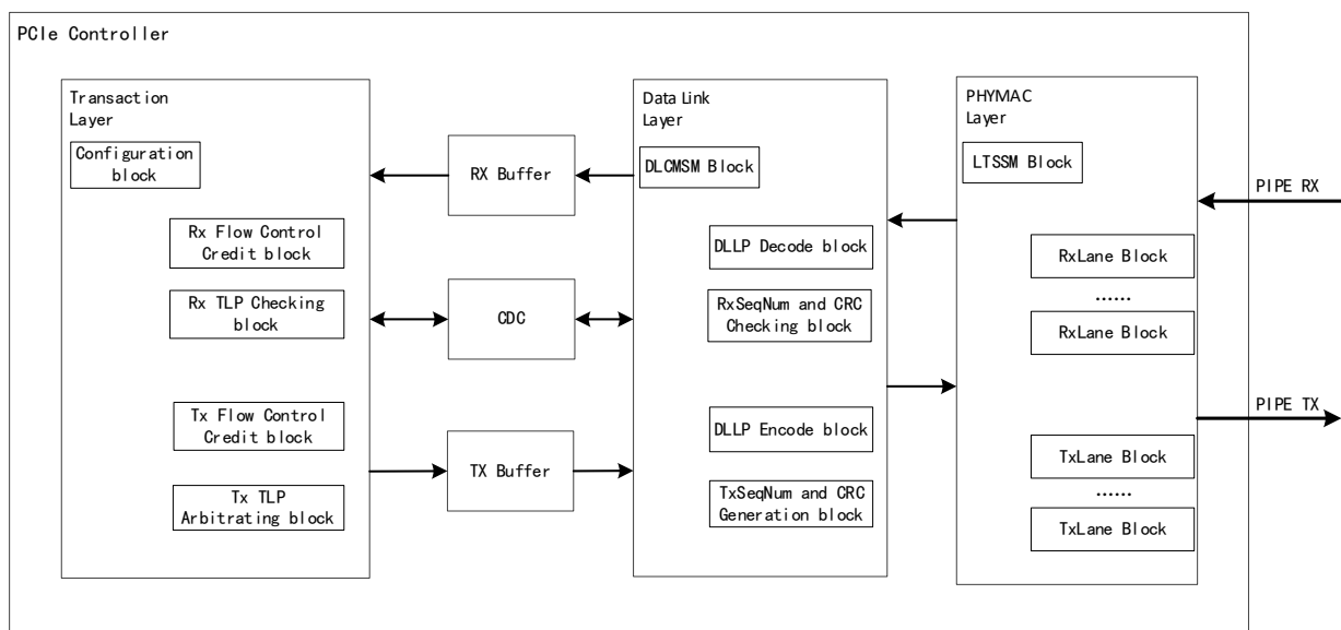
图 1-4 PCI Express 控制器内部框图
