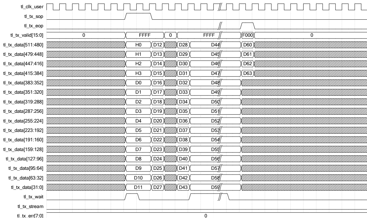
图 2-9 发送 4DW Header With 64DW Payload
