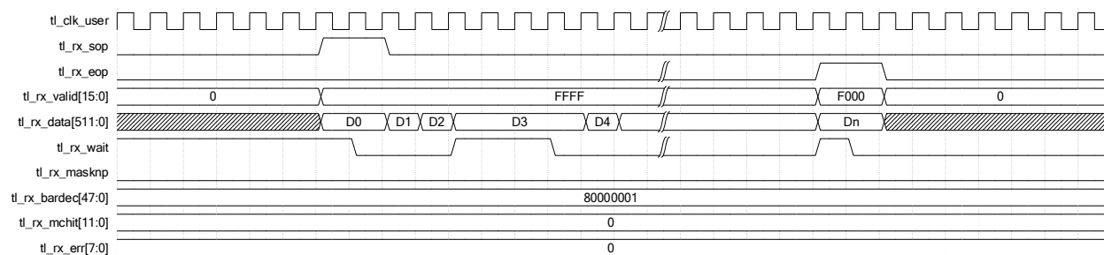
图 2-15 接收过程 wait 信号置 1
