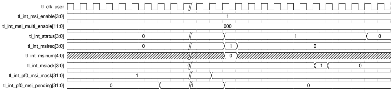
图 2-31 PF0 中断 mask 后重新发送
