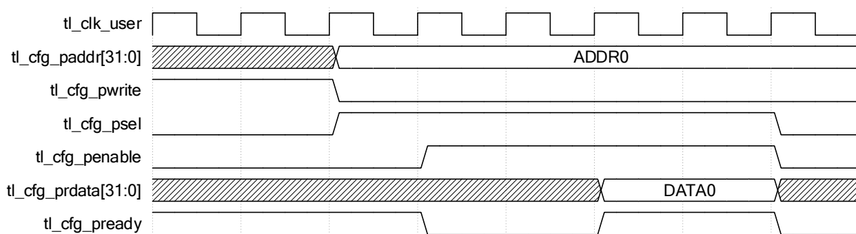
图 2-25 读操作有等待
