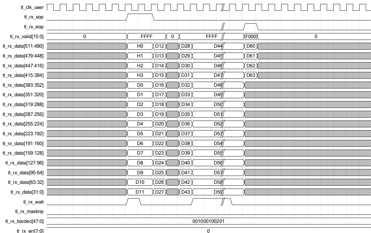
图 2-20 接收 4DW Header With 64DW Payload
