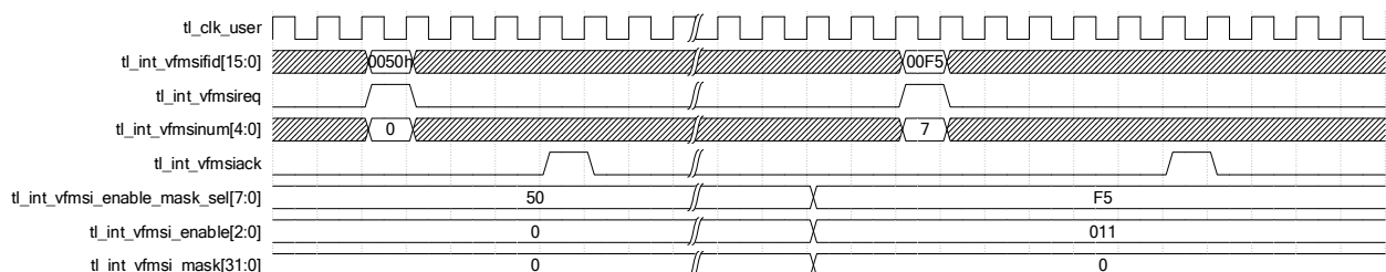
图 2-32 VF 发送 MSI 中断
