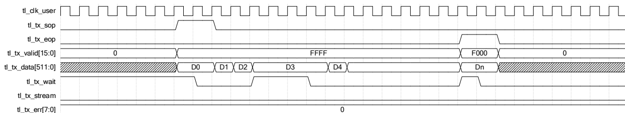
图 2-4 发送过程 wait 信号反压
