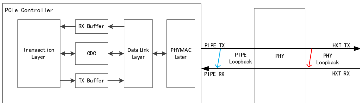
图 3-4 Loopback 的两种方式
