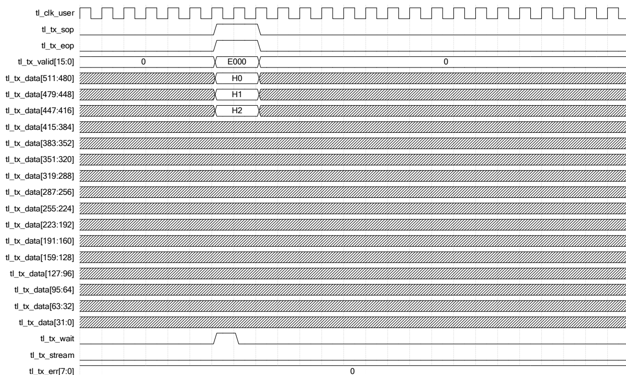
图 2-6 发送 3DW Header Without Payload
