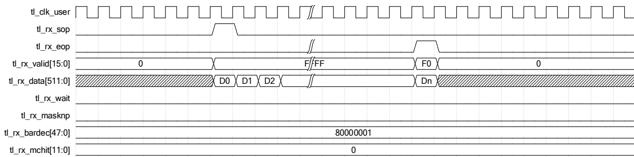
图 2-14 接收过程 wait 信号没有置 1
